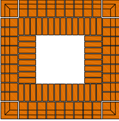
4.sıra planı
