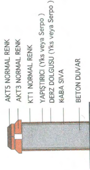
2-2 KESİTİ
