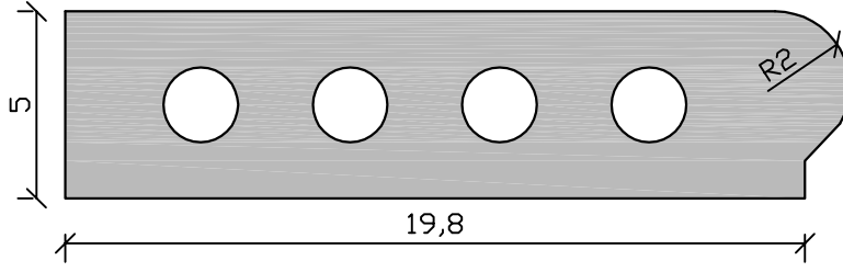
ÖN GÖRÜNÜŞ
