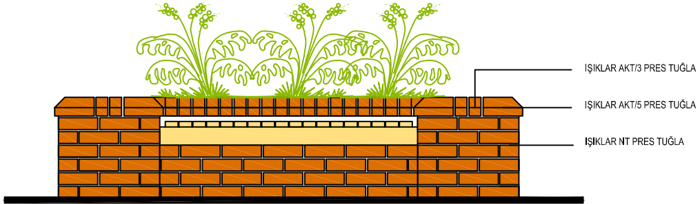
GÖRÜNÜŞ
