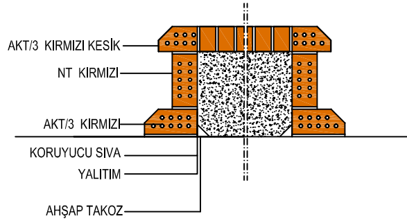
KESİT
