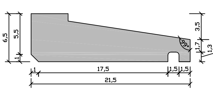
YAN GÖRÜNÜŞ
