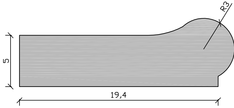
YAN GÖRÜNÜŞ
