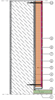
Zemin Detayı
