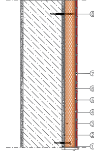
Dikey Kesit
