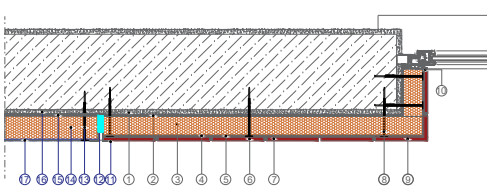
Dilatasyon Birleşim Detayı
