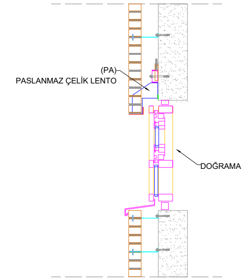
PENCERE DETAYI
