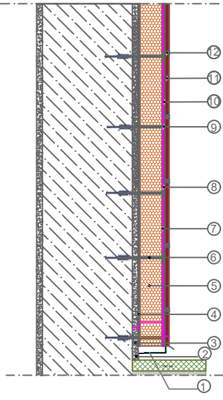
Zemin Detayı
