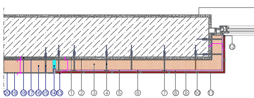
Dilatasyon Birleşim Detayı
