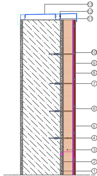
Harpušta Detayı
