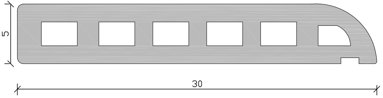
YAN GÖRÜNÜŞ
