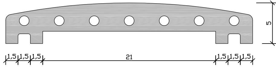
GÖRÜNÜŞ
