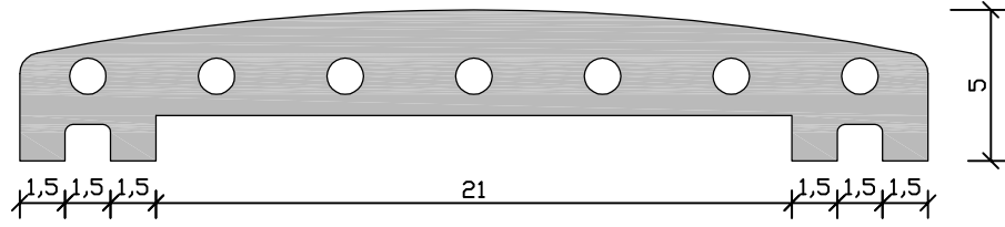
GÖRÜNÜŞ
