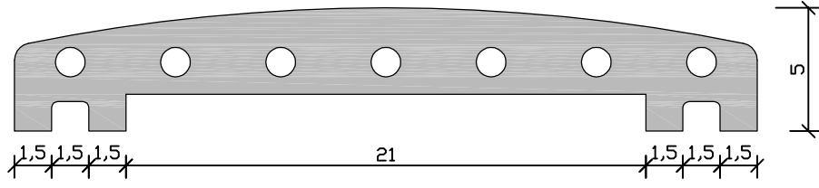
GÖRÜNÜŞ
